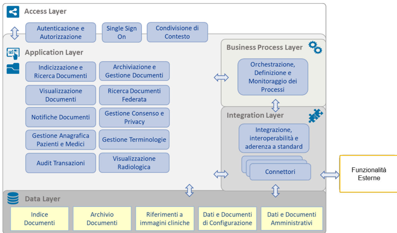
Figura 10 Architettura Funzionale
