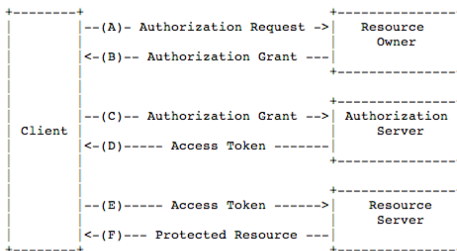
Figura 6- Flusso OAuth2
